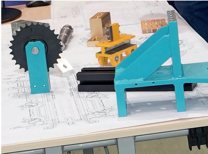
Plan zum Fertigen der Form und fertige Formen
